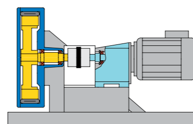
长轴型
