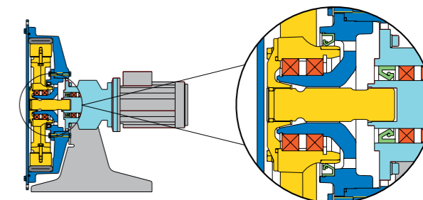
直联式
